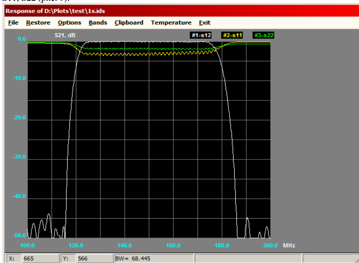
Рис.9. Графики S-параметров.
