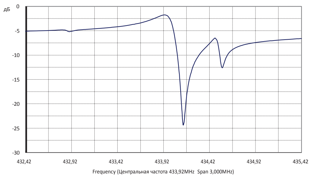
ХАРАКТЕРИСТИКА ПРОХОЖДЕНИЯ |S11|
