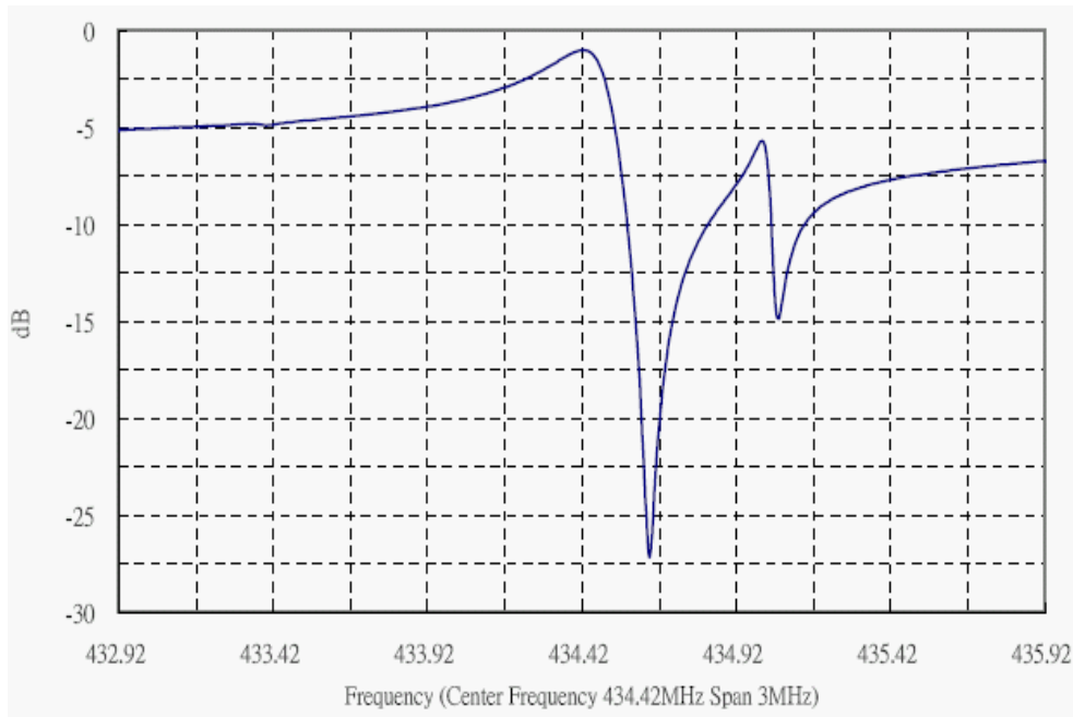
АЧХ
