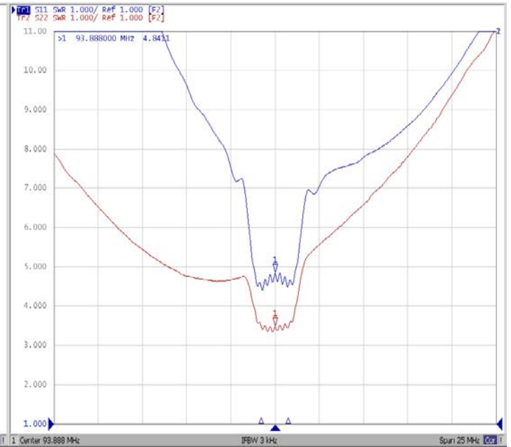
КСВ
