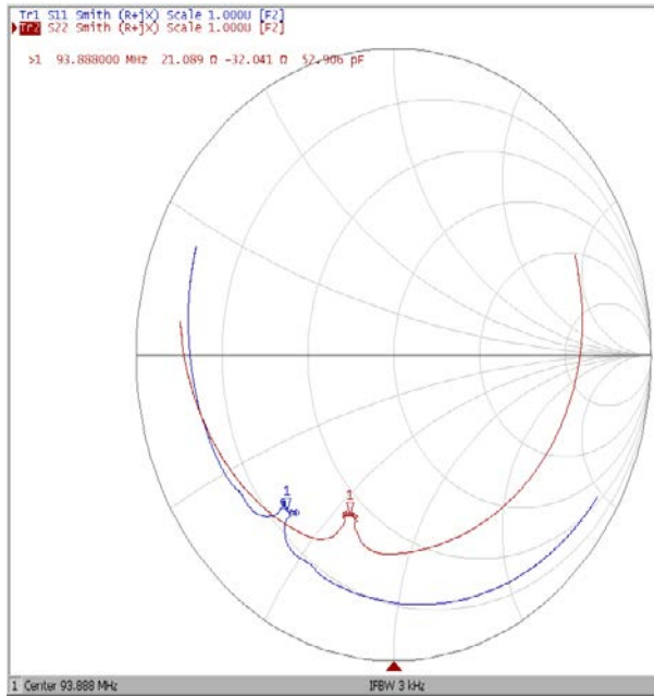
Диаграмма Смита
