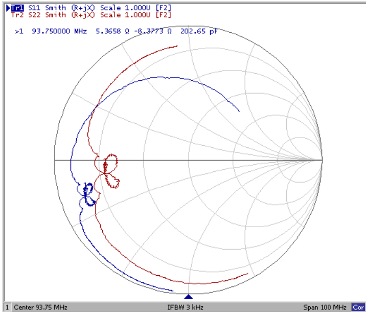
Диаграмма Смита
