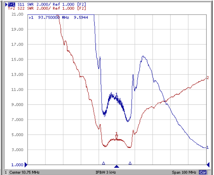
КСВ
