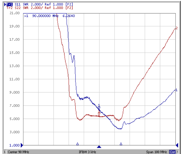
VSWR
