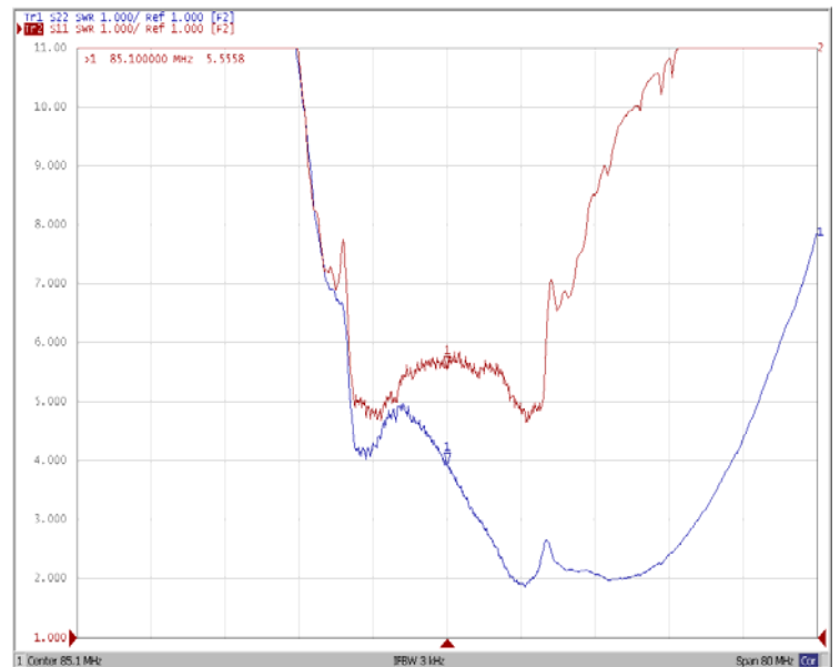
VSWR
