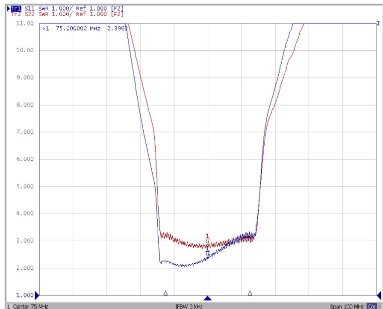
VSWR
