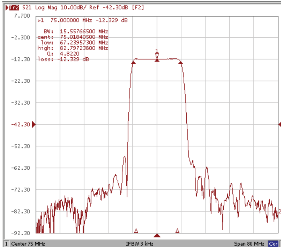
Неравномерность АЧХ в полосе
