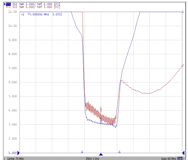
VSWR
