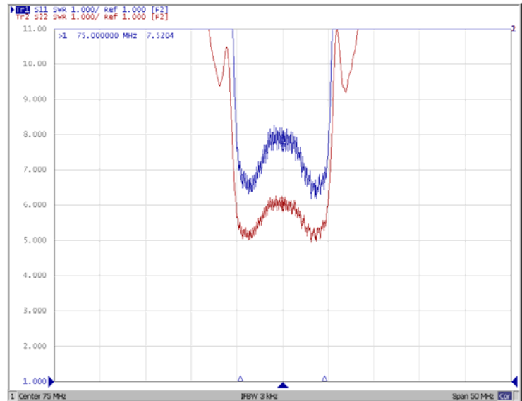
VSWR
