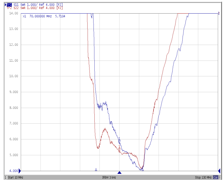
VSWR
