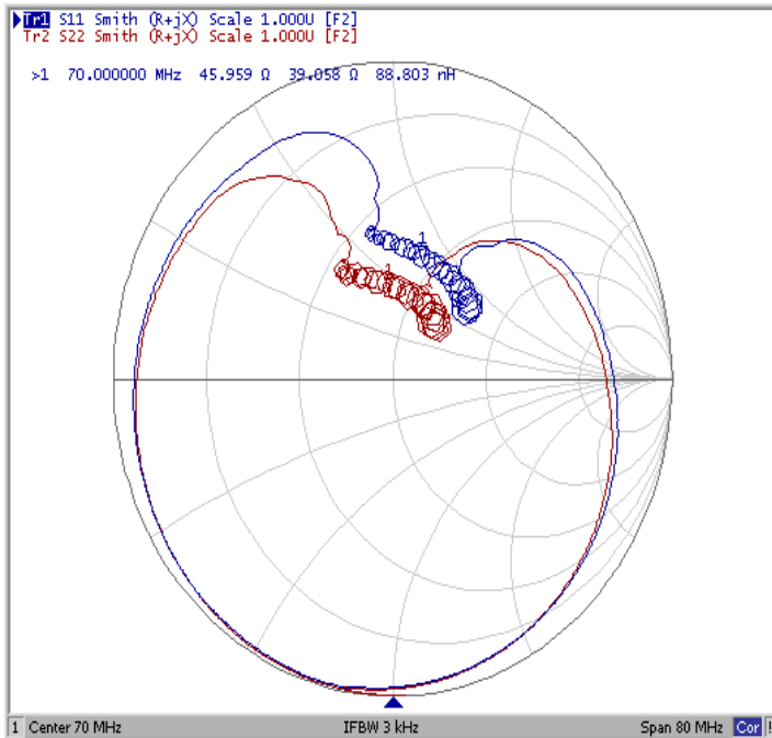
Диаграмма Смита
