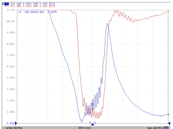
VSWR
