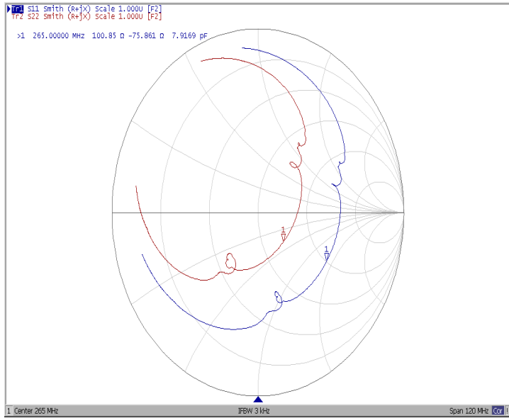
Диаграмма Смита
