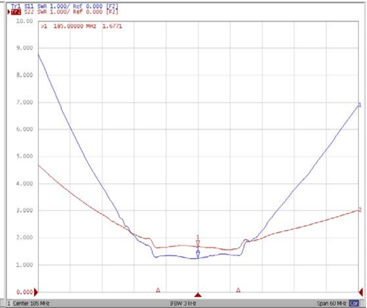
КСВ
