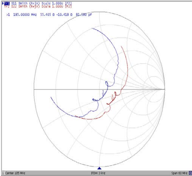
Диаграмма Смита
