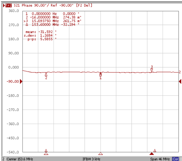
Phase ripple Fo±16.00MHz
