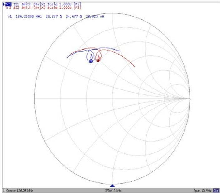
Диаграмма Смита
