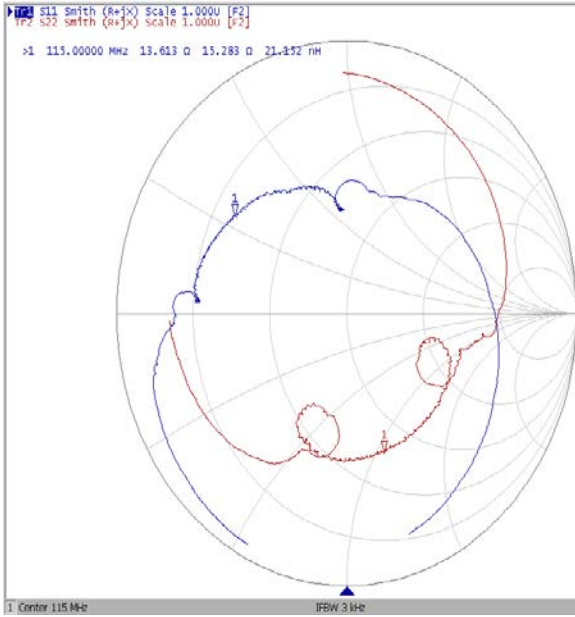
Диаграмма Смита
