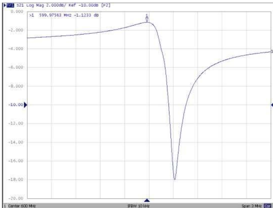
ХАРАКТЕРИСТИКА ПРОХОЖДЕНИЯ |S11|
