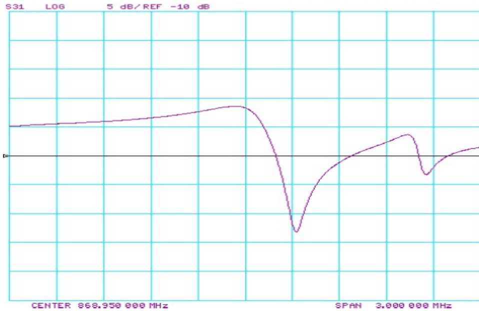
АЧХ
