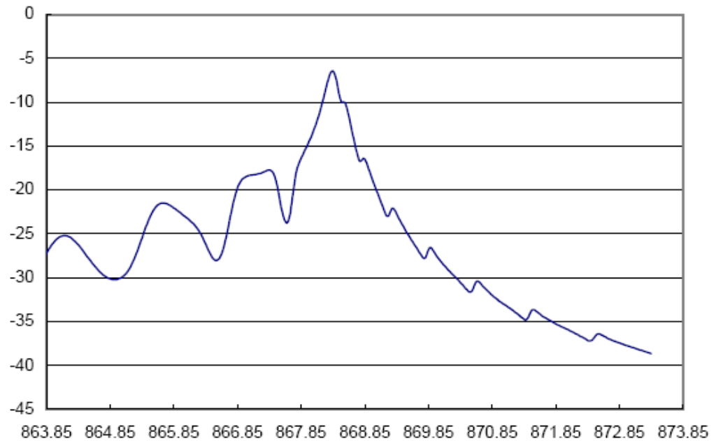
АЧХ
