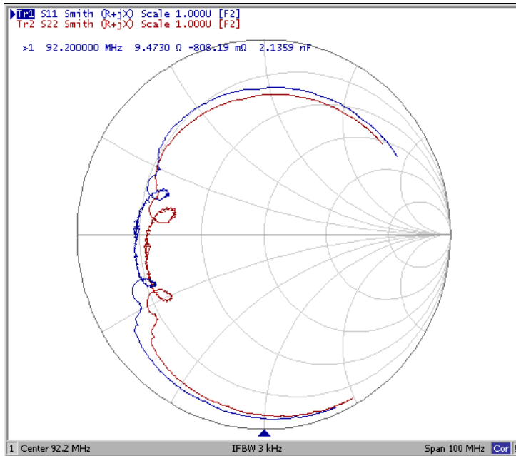
Диаграмма Смита
