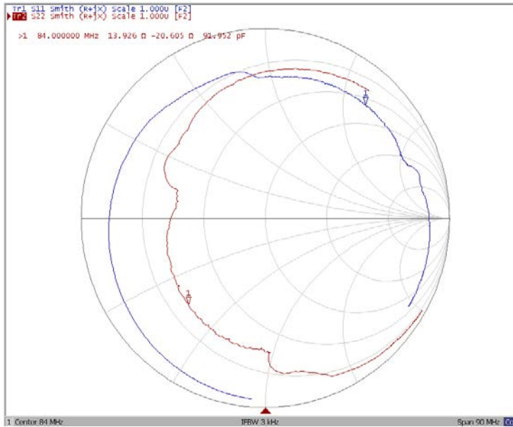
Диаграмма Смита
