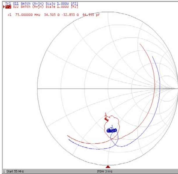
Диаграмма Смита
