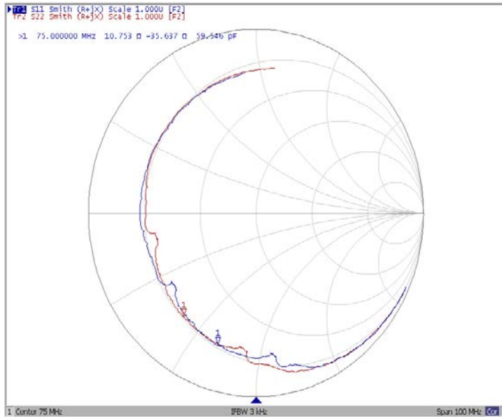
Диаграмма Смита
