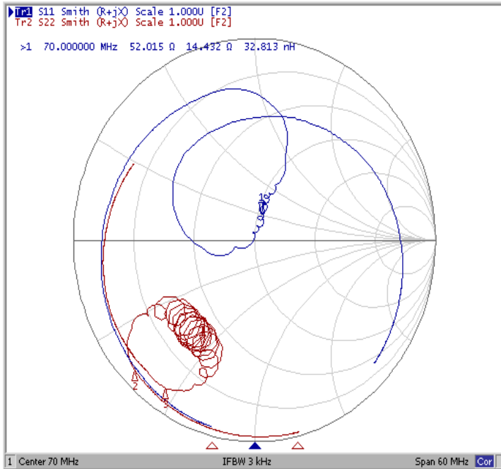
Диаграмма Смита
