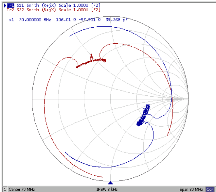
Диаграмма Смита
