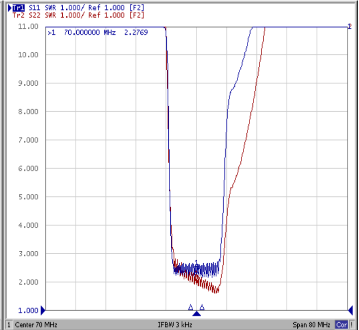
КСВ
