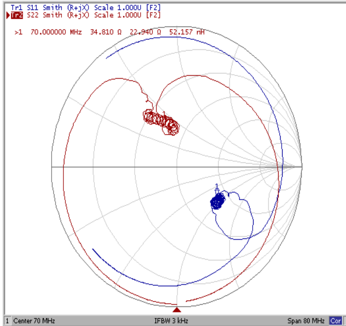
Диаграмма Смита
