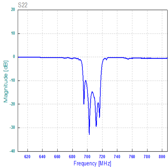
Потери на отражение S22, дБ
