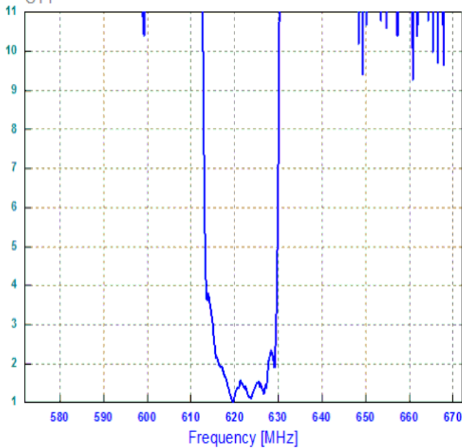
КСВ S11
