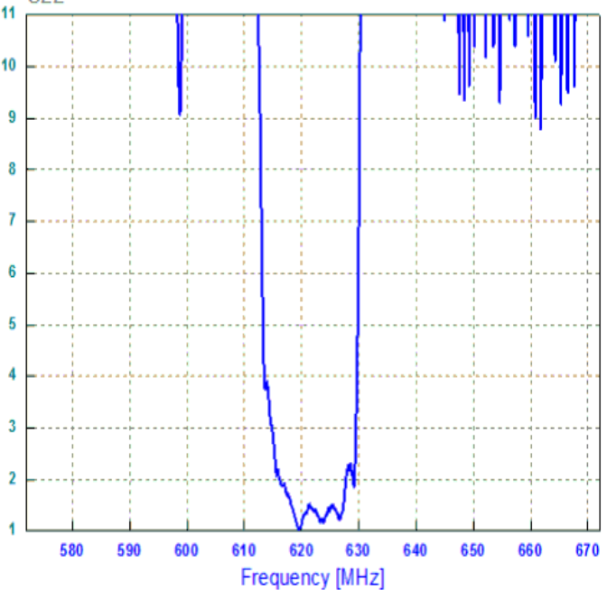
КСВ S22
