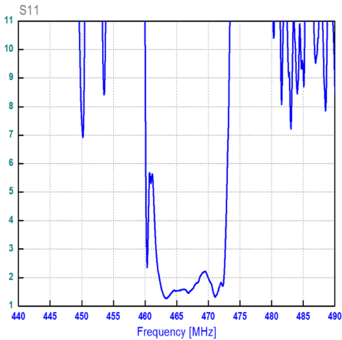
КЧВ S11
