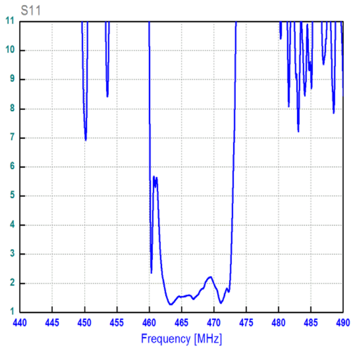
КСВ S11
