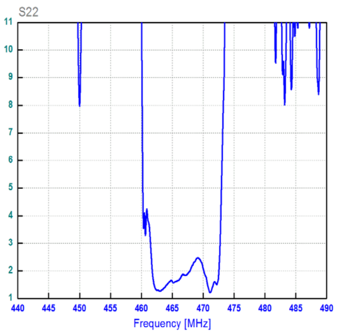
КЧВ S22
