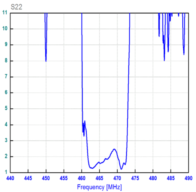
КСВ S22
