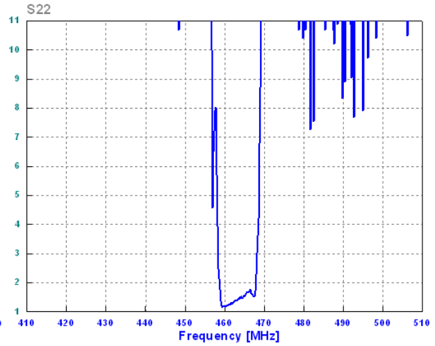
КСВ S22
