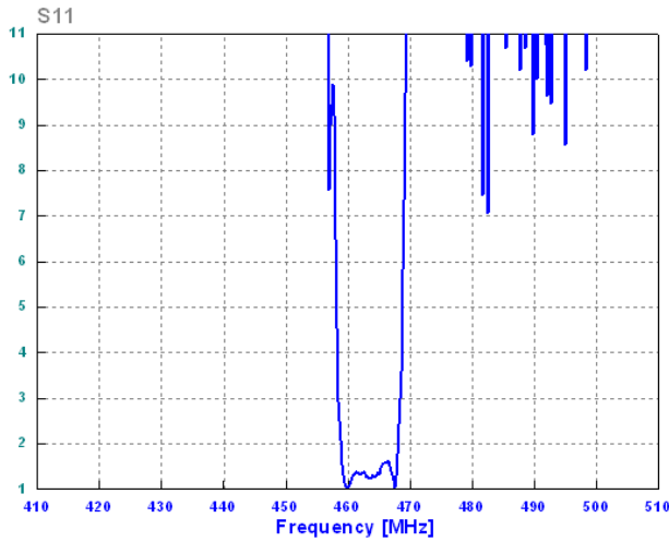
КСВ S11
