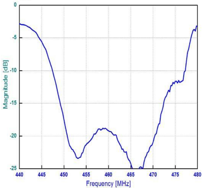
Потери на отражение S11, дБ
