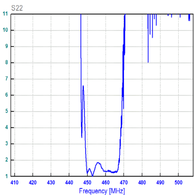
КСВ S22
