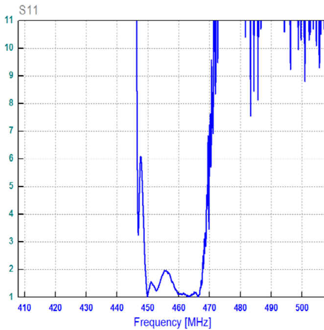
КСВ S11
