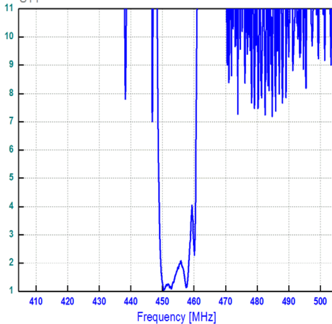
КСВ S11
