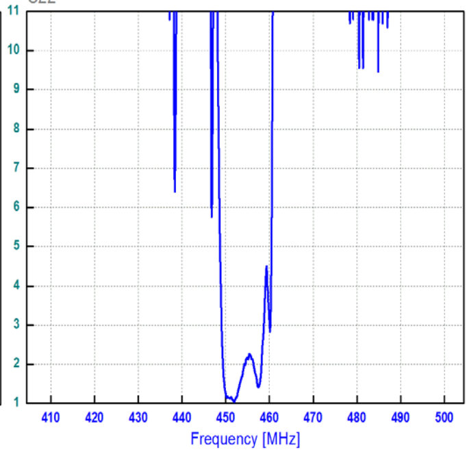
КСВ S22
