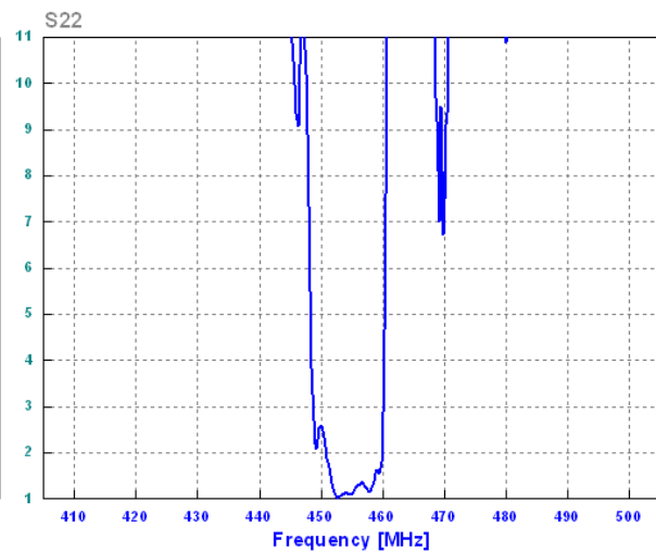
КСВ S22
