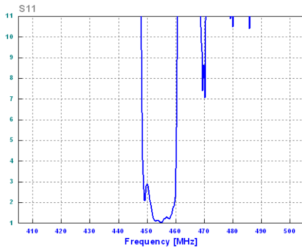
КСВ S11
