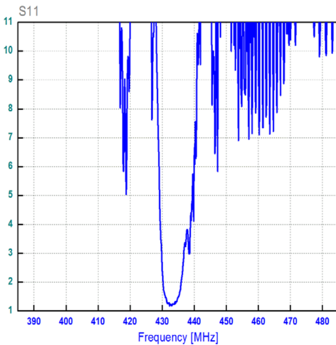
КСВ S11
