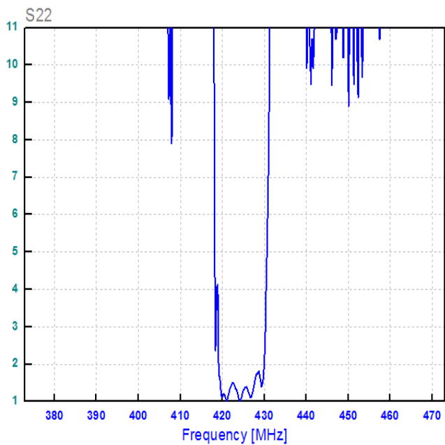
КСВ S22
