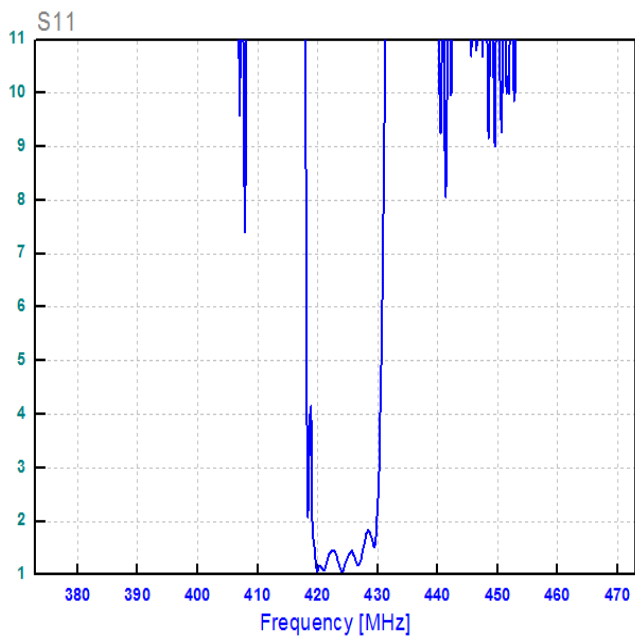
КСВ S11
