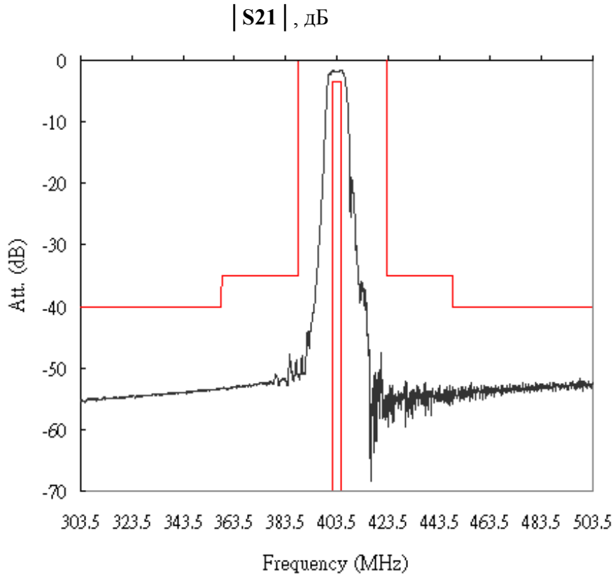
|S_{21}| , дБ (393,5 МГц~ 413,5 МГц)
