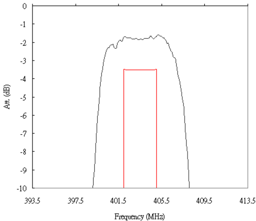
|S_{21}| , дБ (393,5 МГц~ 413,5 МГц)
