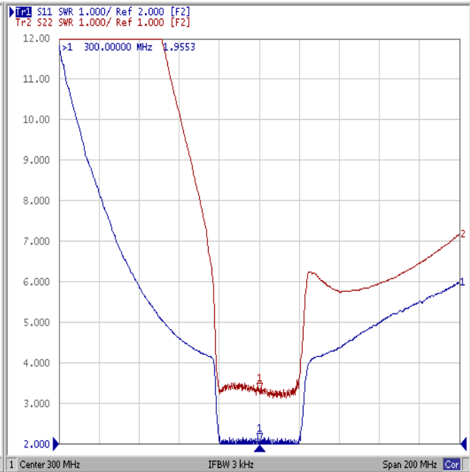
КСВ
