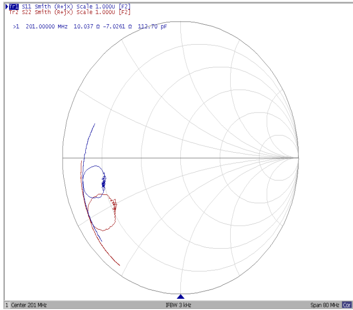
Диаграмма Смита
