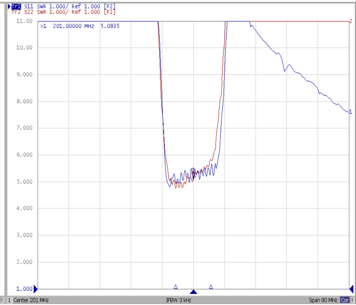
КСВ
