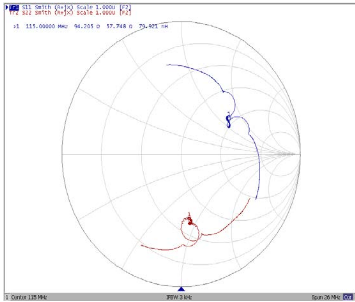
Диаграмма Смита
