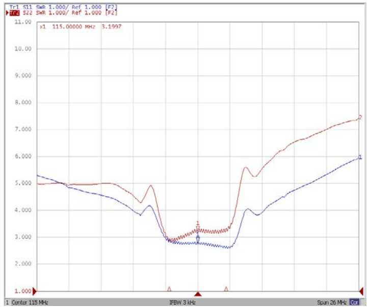
КСВ
