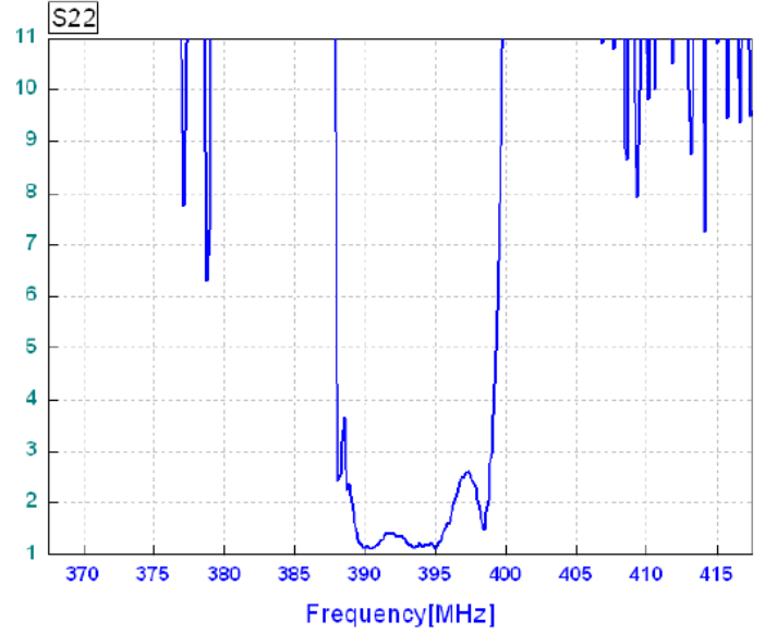
КСВ S11
