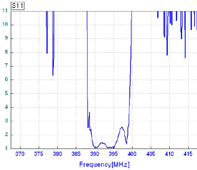
КСВ S11
