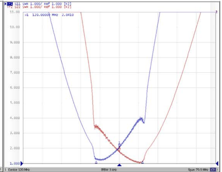
КСВ
