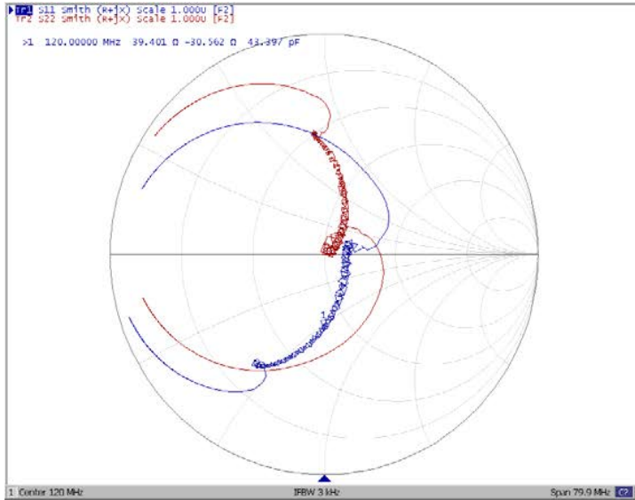
Диаграмма Смита
