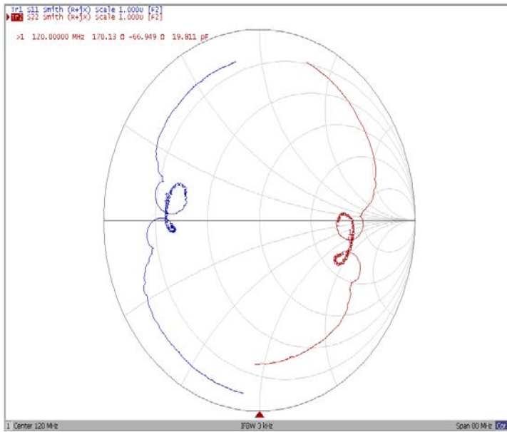
Диаграмма Смита
