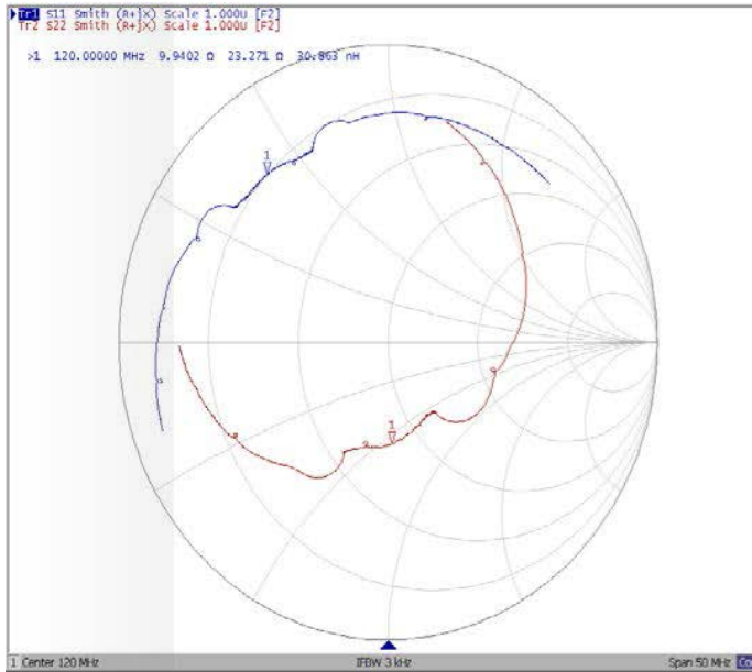
Диаграмма Смита
