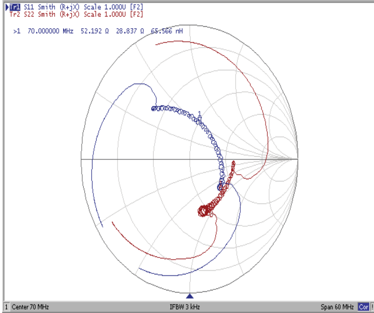
Диаграмма Смита
