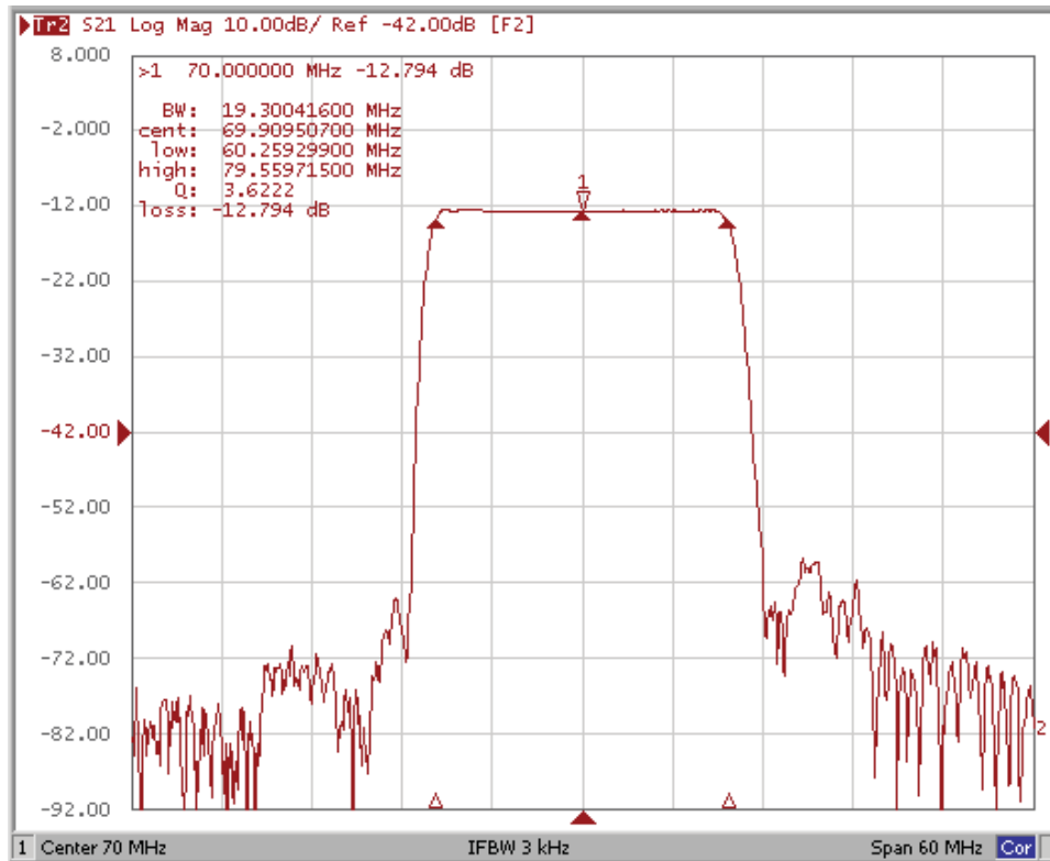
Неравномерность АЧХ в полосе
