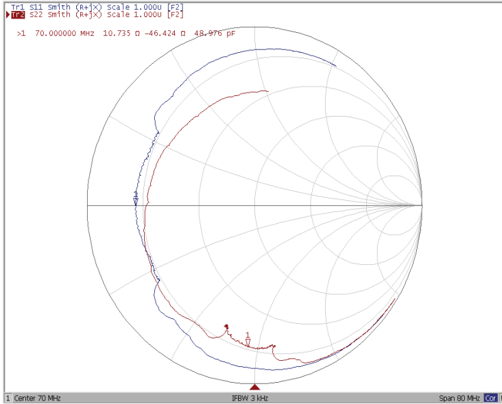
Диаграмма Смита
