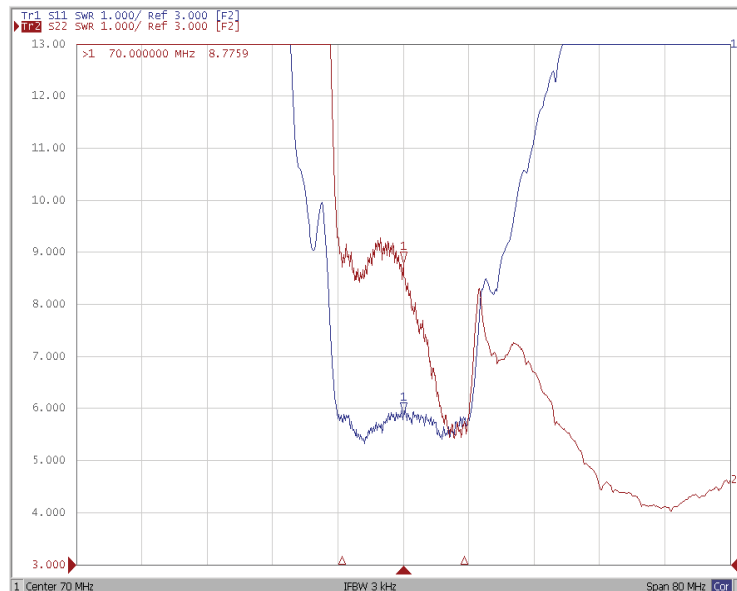
КСВ
