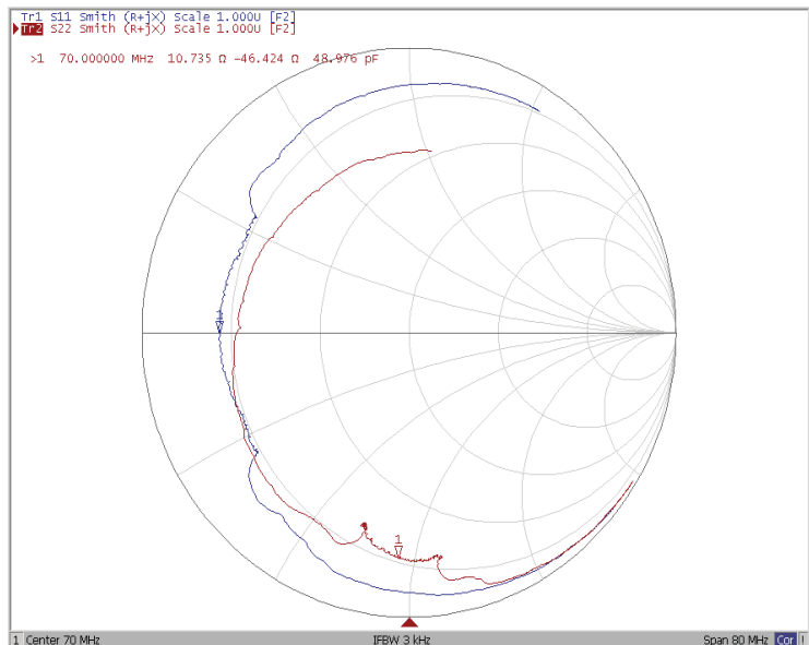
Диаграмма Смита
